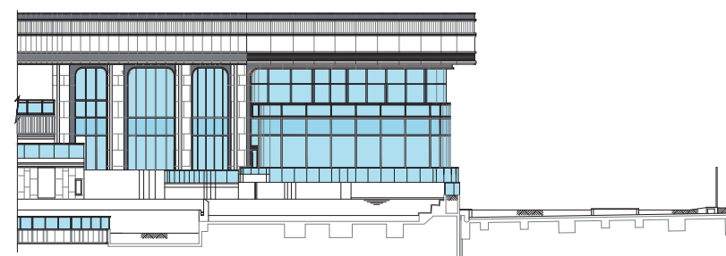
立面圖 7 Elevation Plan 7
